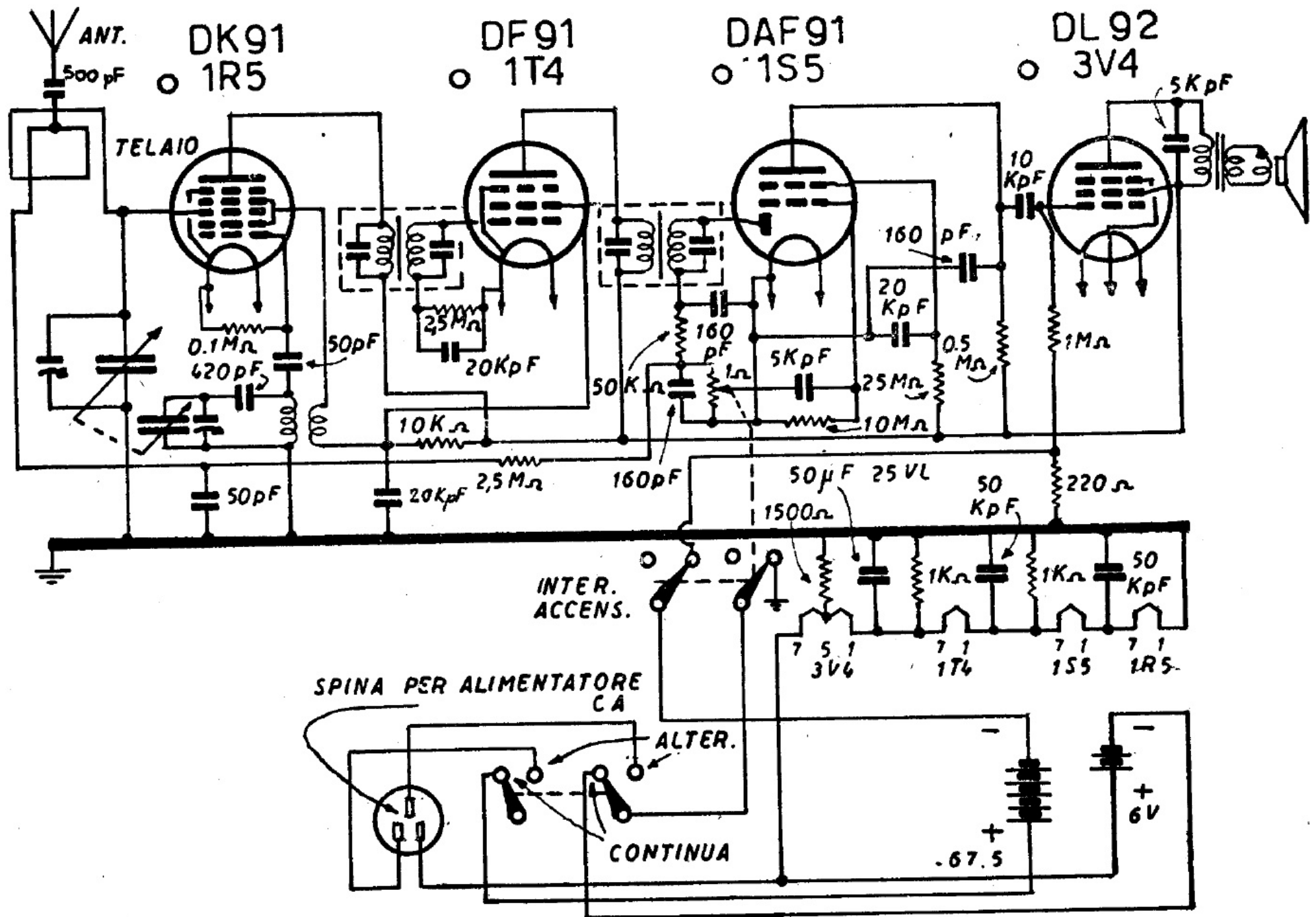
NOVA RADIO - Portatile a pile mod. E.1 - Medie 187-582 metri. Media frequenza 465 kc. Batterie: Minimicro 6 V per accensione, Mini-micro 67,5 volt per anodica. Alimentatore separato per CA 110/125 volt.
